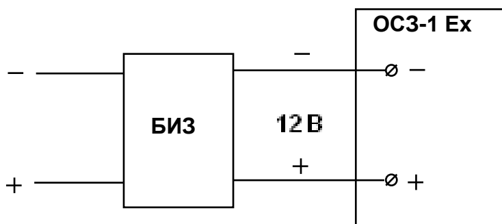
Рис.3 Пример подключения оповещателя во взрывозащищенном исполнении OC3-1 Ex.
