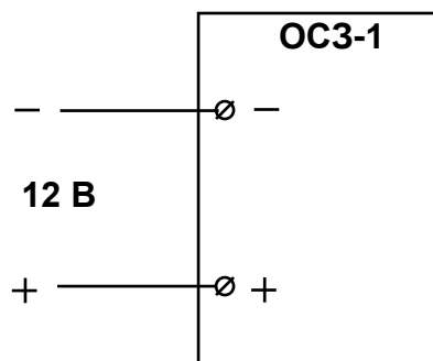
Рис.2 Пример подключения оповещателя OC3-1.
